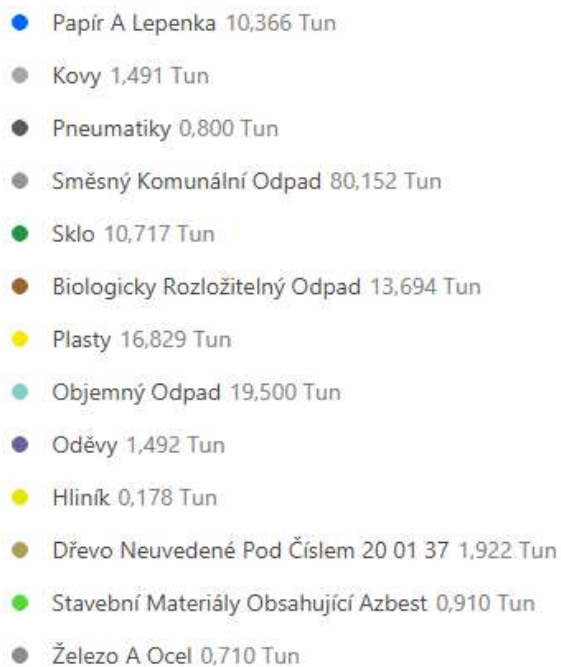
Sumarizační graf
